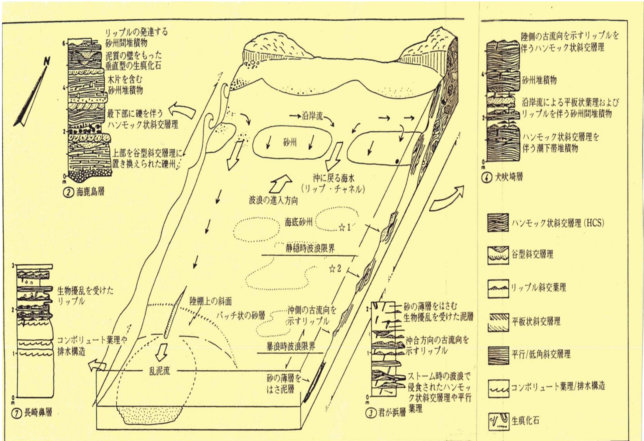
☆1 ハンモック状斜交層理と陸側の古流向を示すリップル ☆2 ハンモック状斜交層理と沖側の古流向を示すリップル
